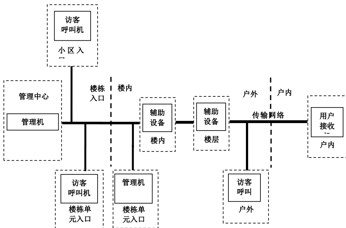
图 4 楼宇对讲系统应用构成示意图
