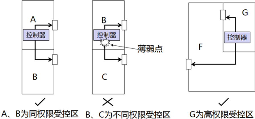
图2 出入口控制系统受控区的设备安装示意图
